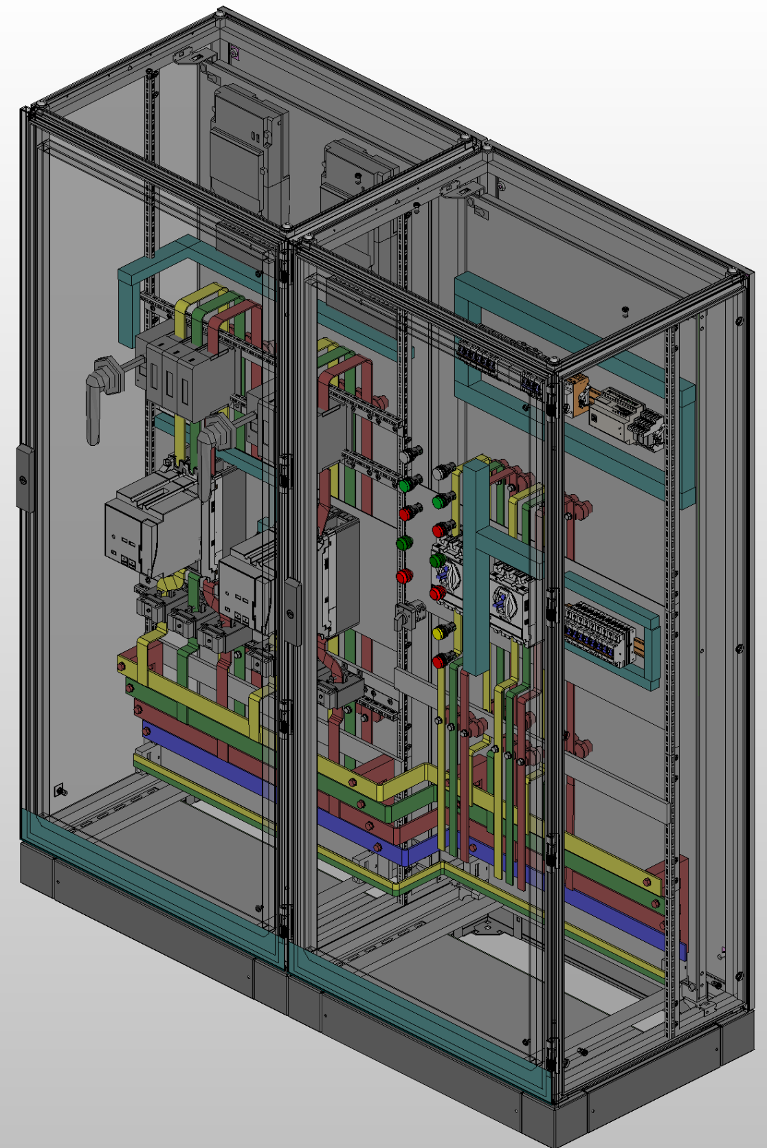
Вид спереди с дверями (изометрия)
